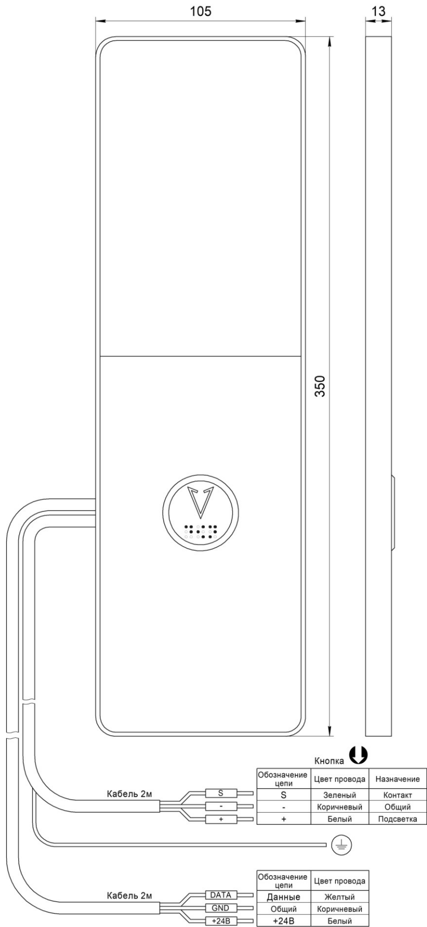
Рис.1 Внешний вид, габаритные и установочные размеры Вызывного поста GOLD НШЕК.468381.201-01
